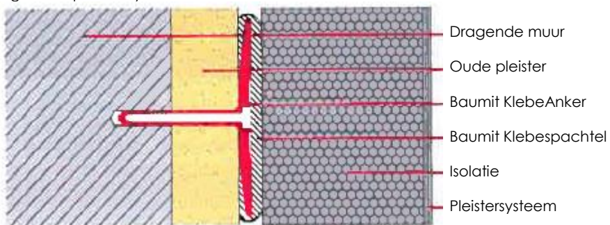
Figuur 2: opbouw systeem - dwarsdoorsnede
